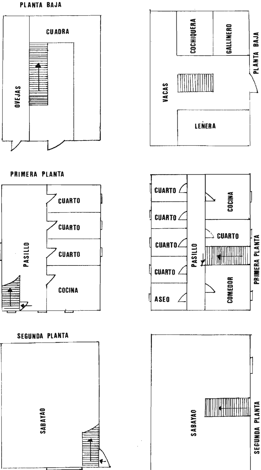
Plano de una borda
