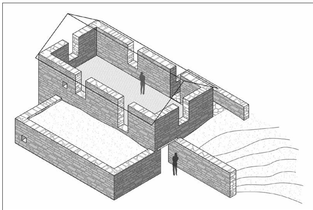
Figura 5. Reconstrucción de la Estructura II, una tipología germana de construcción. La figura 4 es una foto de la puerta inferior de esta estructura.
