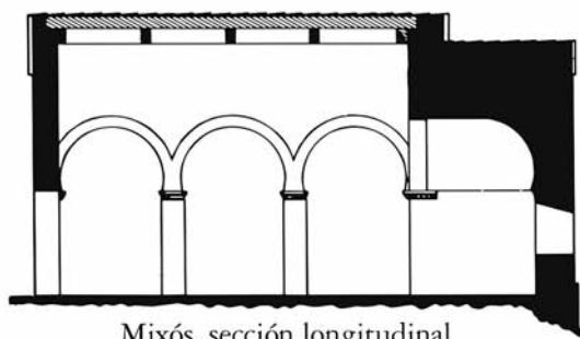
Mixós, sección longitudinal
