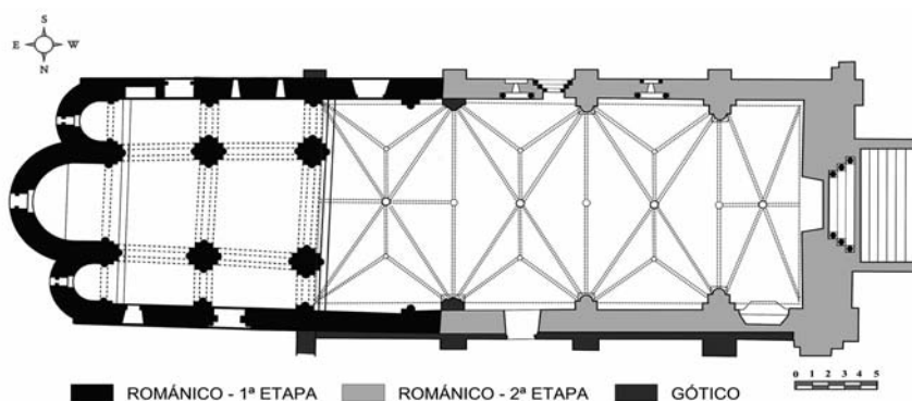
Fig. 11. Planta de la iglesia actual, según Fco. Javier Ocaña Eiroa
