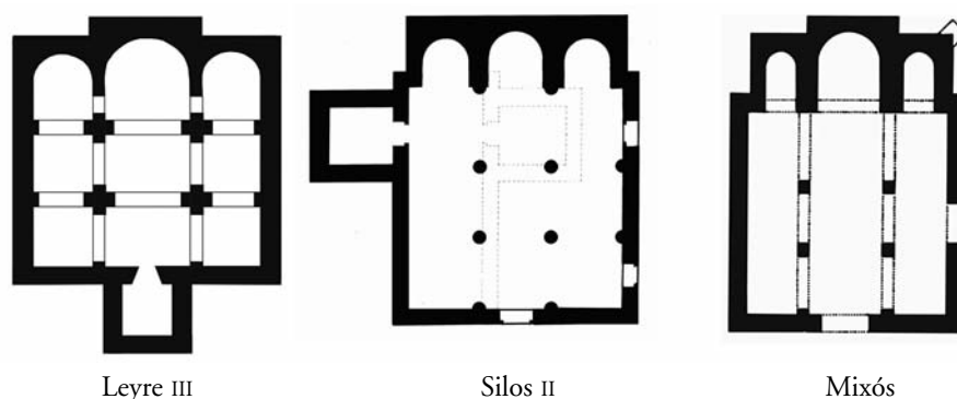
Fig. 6. Comparación de plantas mozárabes de una sola nave con crucero
